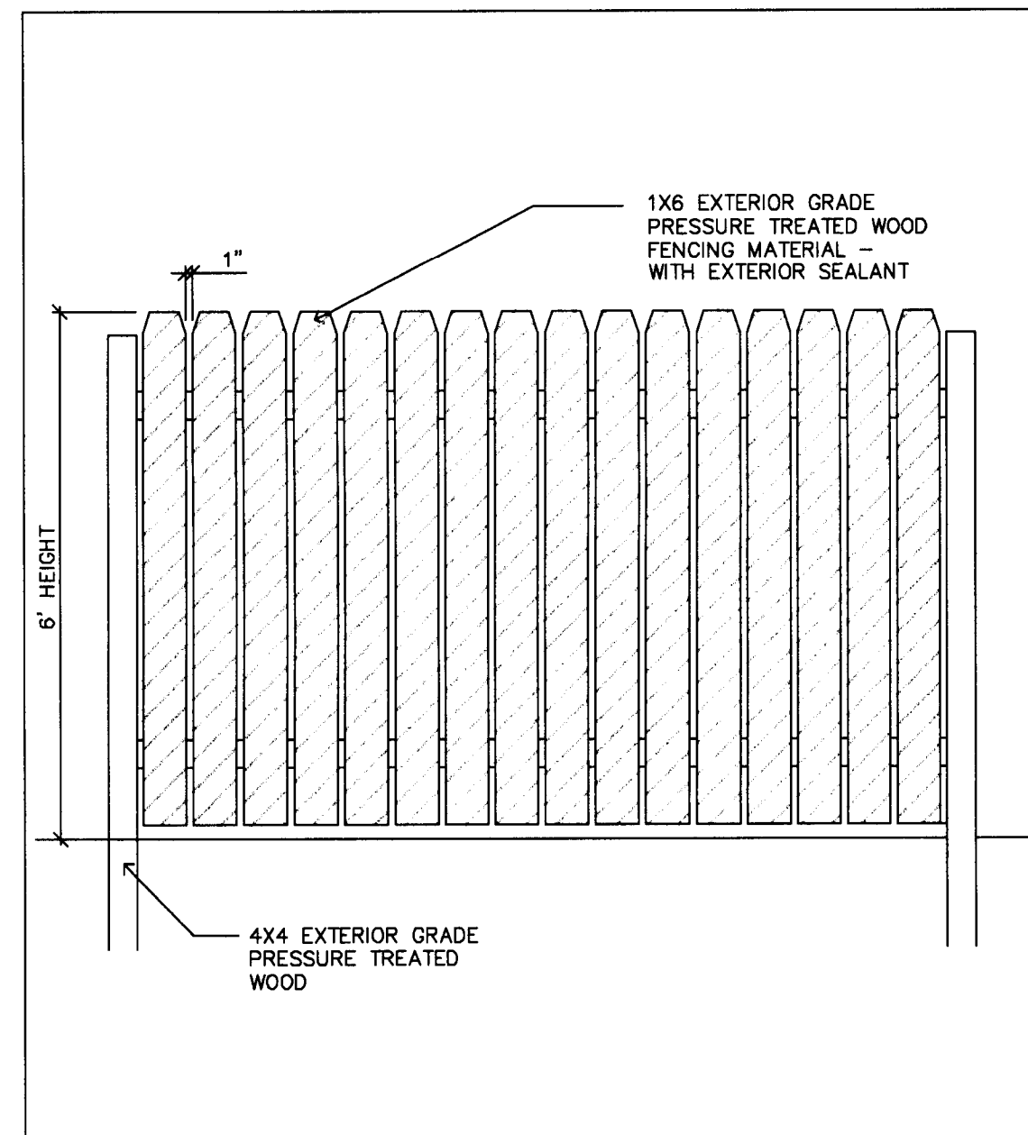
FENCE DETAIL N.T.S. 4
